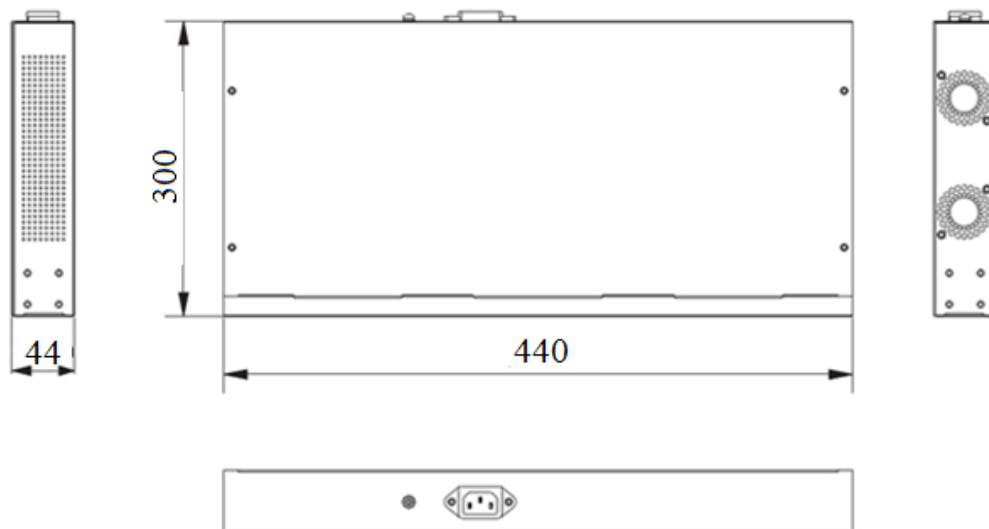
Рисунок 4.2 Габаритные размеры
