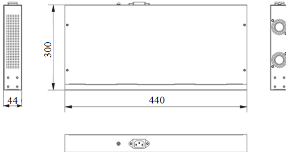
Рисунок 4.3 Габаритные размеры
