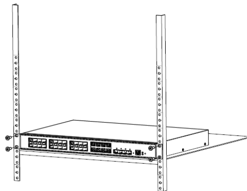
Рисунок 4.4 Монтаж
