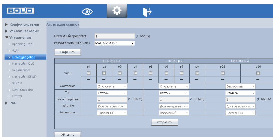
Рисунок 7.21 Интерфейс настройки агрегации ссылок
