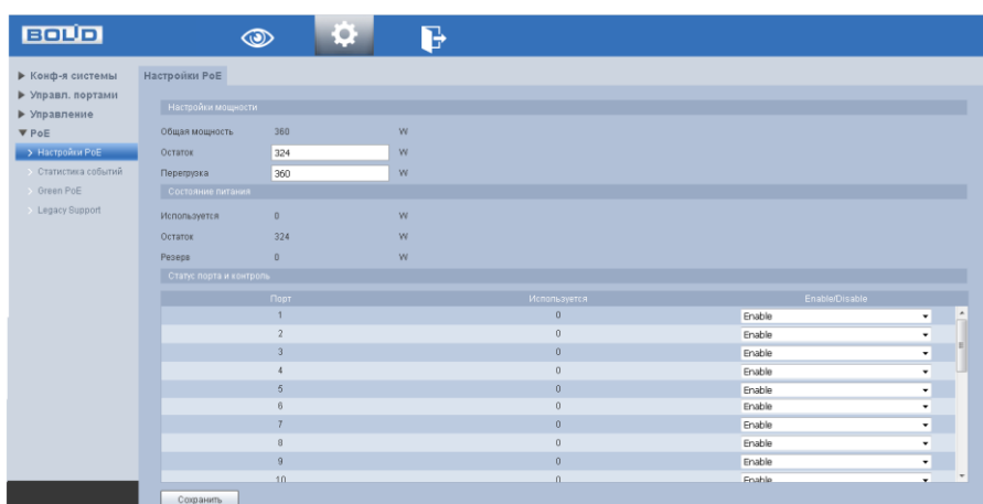
Рисунок 7.37 Питания порта по PoE
