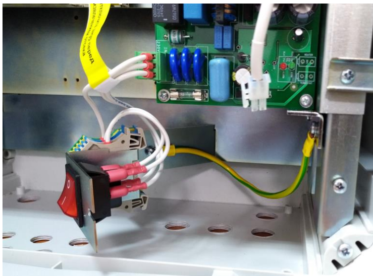
Рисунок 3.5.2 – Узел подключения питания освобожден от крепежа.
