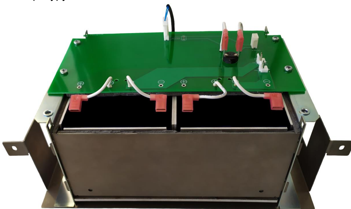
Рисунок 3.9 – АКБ отсек.
