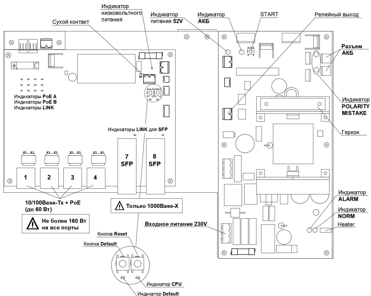
Рисунок 3.4.2 – Расположение элементов PSW-2G+UPS-Box
